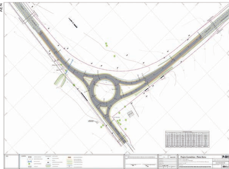
Planta mostra como ficará o trevo que dá acesso aos dois balneários na Costa Noroeste
