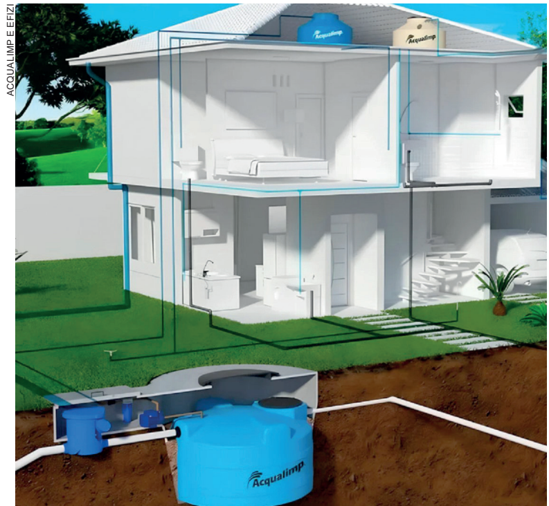
Ilustração de instalação de cisterna em edificações
